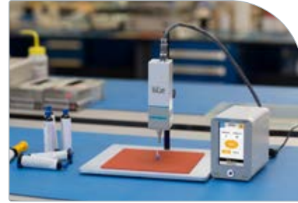
BlueWave® MX-150™ LED点光源固化系统
